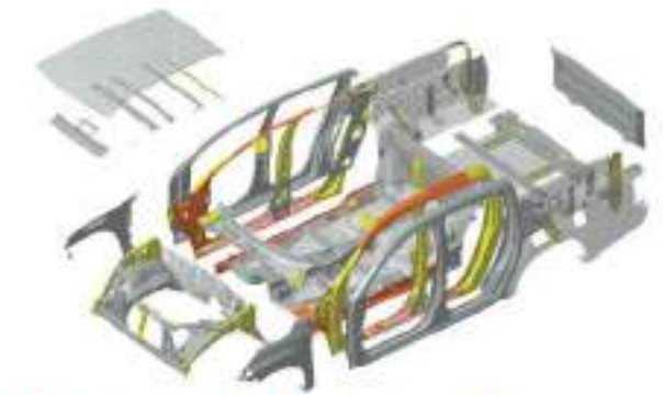
■ 980Mpa class ■ 590Mpa class ■ 440Mpa class
